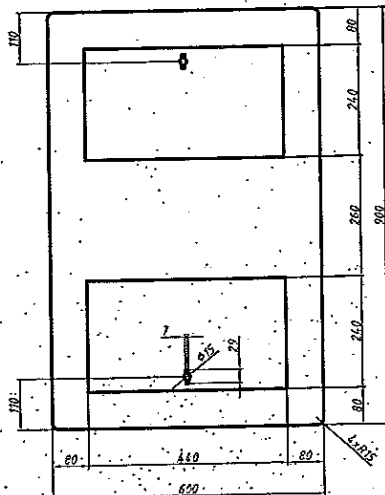
Капак за ЕЛЕКТРОШАХТИ поглед от долу
