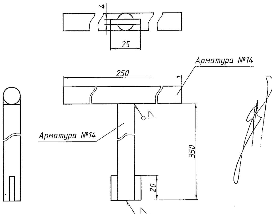
Инструмент за повдигане на капак за електрошахти
