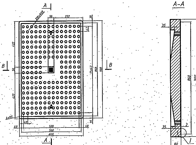
Капак за ЕЛЕКТРОШАХТИ поглед отгоре
